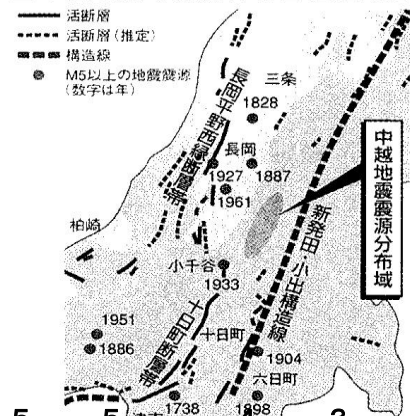
■ 中越地震の震源分布図と活断層
